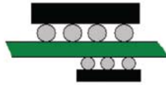
Рис. 23. Недопустимое расположение компонентов BGA один над другим
